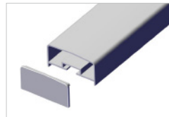
Handlauf 75x38 mm für teilflächige Füllungen
