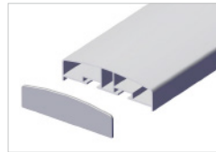
Handlauf 137x38 mm für vollflächige Füllungen
